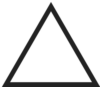
oblik trokuta
